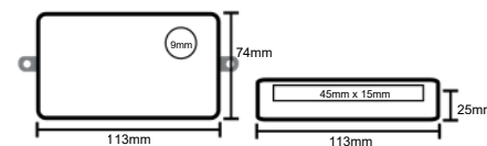
Módulo SW - Cód.: 1368 Tampa inferior
