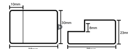
Gabinete Impacto fechado - Cód.: 1667 Tampa inferior
