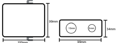
Gabinete standart - Cód.: 1491 Tampa frontal 2 furos
