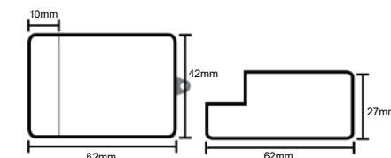
Módulo SW - Cód.: 1368 Tampa inferior
